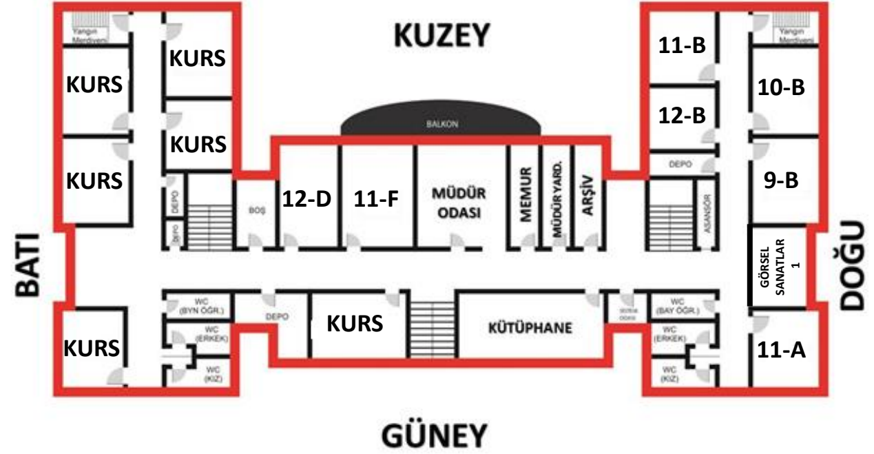
3. KAT PLANI
